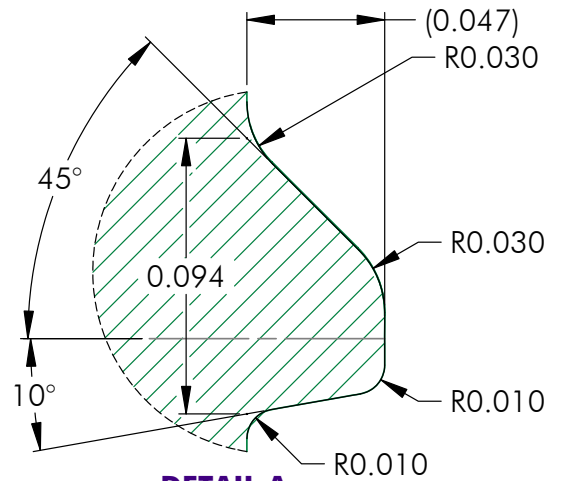
DETAIL A SCALE: 16 : 1
